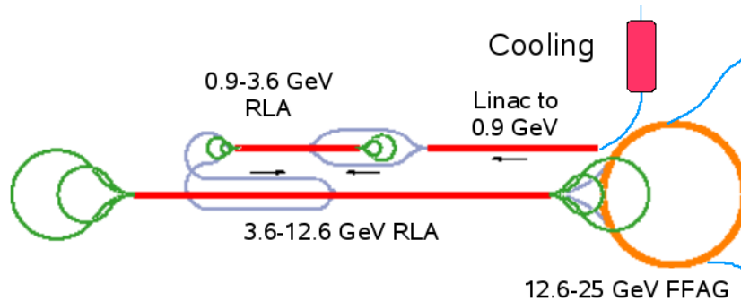
Fig. 7. IDS-NF Baseline acceleration scenario.
