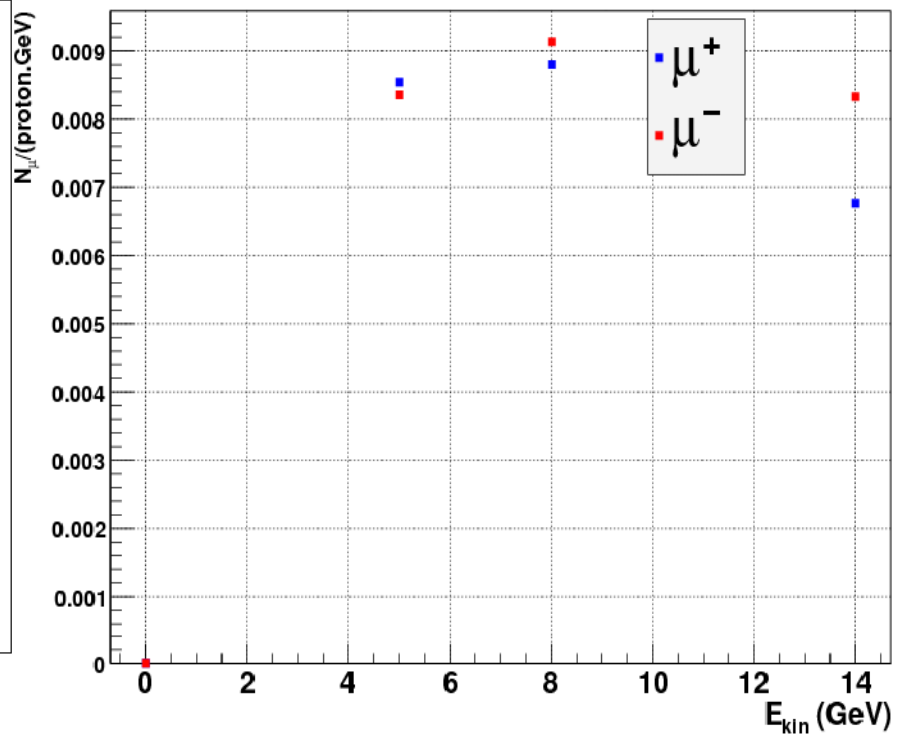
Muon yield per proton and per GeV - ST2a
