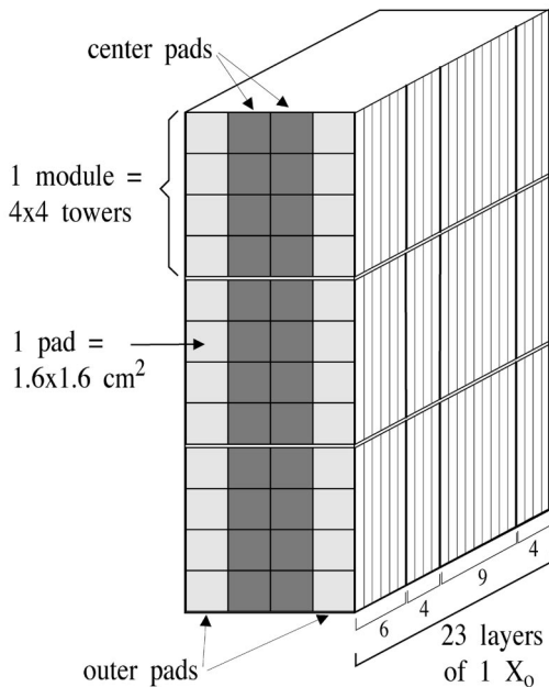
FIG. 17. The electron calorimeter (ECAL).
