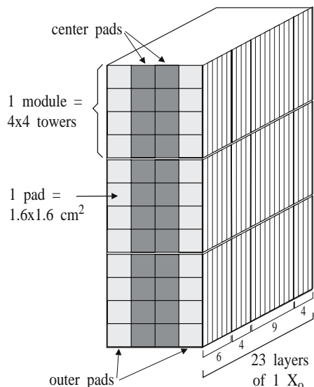
FIG. 17. The electron calorimeter (ECAL).
